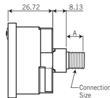
Dimensions Data
